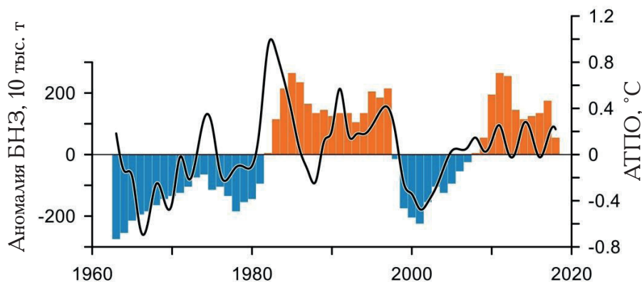
Рис. 7. Динамика аномалий биомассы нерестового запаса минтая северной части Охотского моря (БНЗ, столбики) и средних зимних аномалий температуры поверхности Охотского моря (АТПО, линия).
