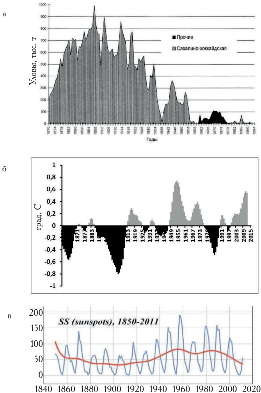
Рис. 15. Вылов сахалино-хоккайдской сельди (а); динамика АТПО, сглаженная 11-летним скользящим осреднением, в районе Куроисио-Ойясио в январе—апреле 1854—2017 гг. (б); количество солнечных пятен (голубая линия) и вековые колебания солнечной активности (1860—1945 и 2010—2070 гг.) (красная линия) (Второй оценочный..., 2014) (в).
