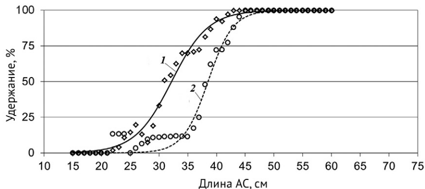
Рис. 1. Графики селективности капроновых траловых мешков с внутренним размером ячеи 100 мм: 1 – без селективной вставки; 2 – с селективной вставкой
