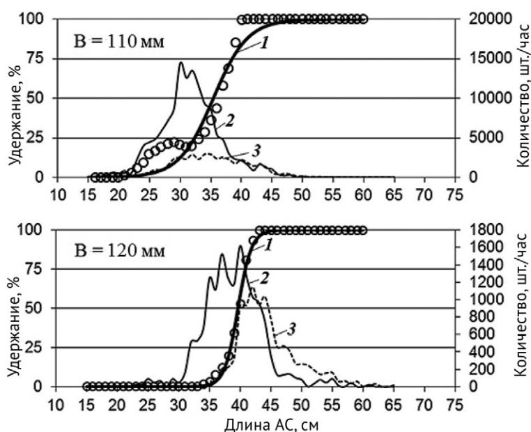
Рис. 2. Графики селективности траловых мешков из мононити с различным внутренним размером ячейи (В) и размерный состав уловов контрольного и экспериментального мешков: 1 – кривая селективности; 2 – размерный состав уловов контрольного мешка; 3 – размерный состав уловов экспериментального мешка
