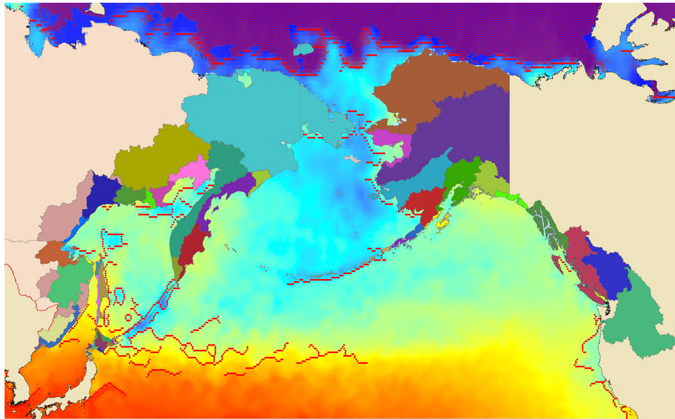
Фронтальные зоны (градиент 1^{\circ}\text{C} и более) на 27 июля 2025 года
