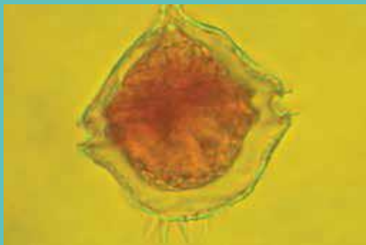
Peridinium trochoideum
