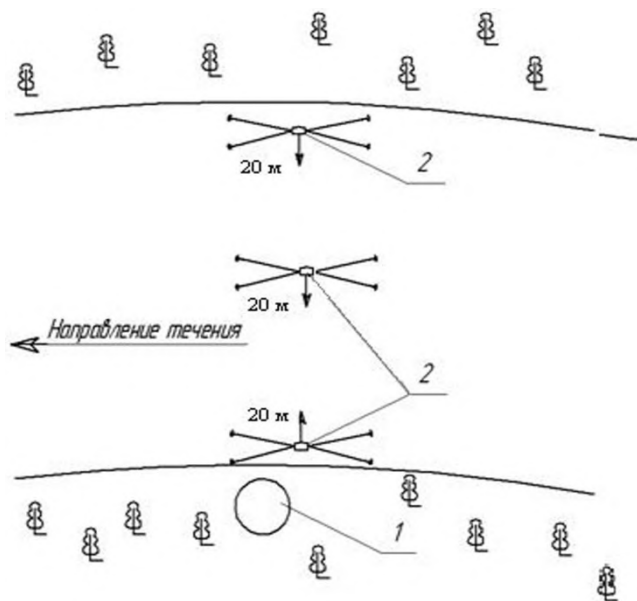
Рис. 1. Схема установки гидроакустических станций комплекса «NetCor» в р. Озерная: 1 — береговая контрольно-измерительная станция; 2 — плавучие гидроакустические станции
