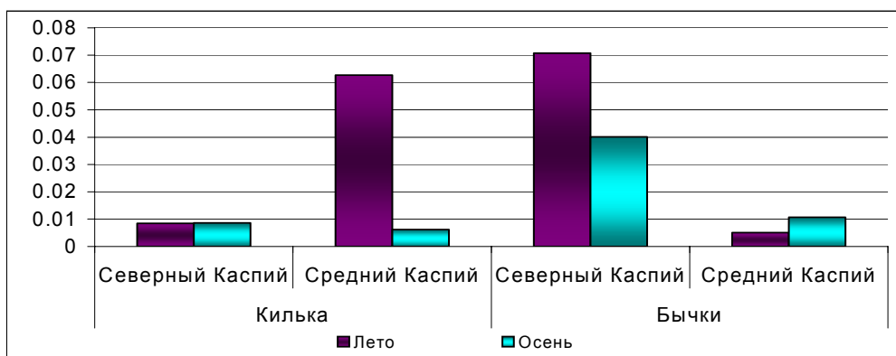
Рис. 1. Содержание ртути в органах и тканях обыкновенной кильки и бычков-песочников мг/кг
